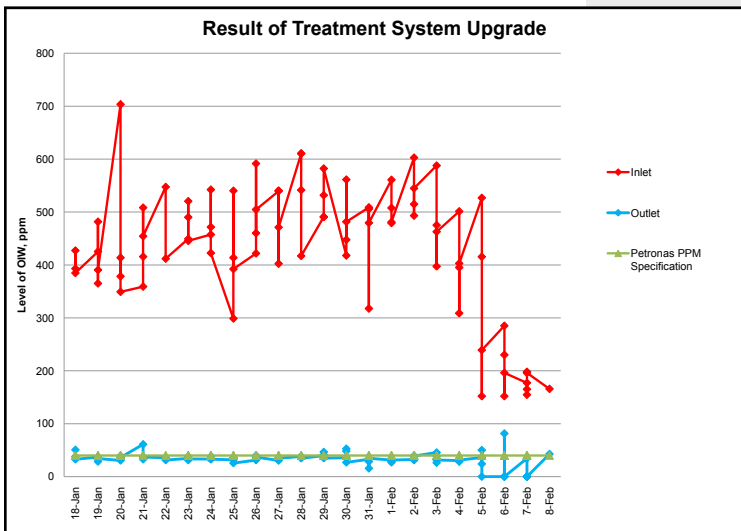
48" CrudeSep
